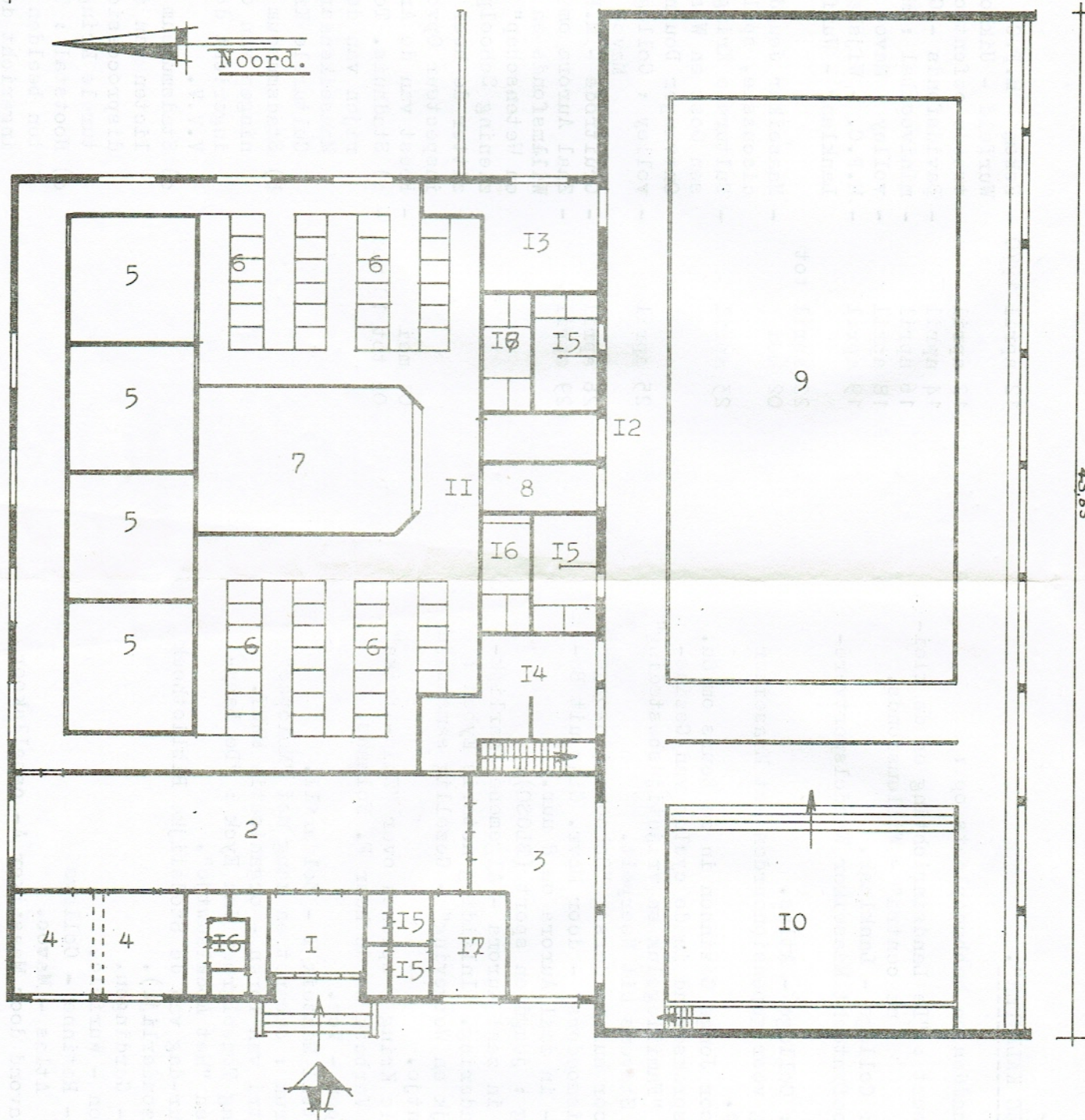
INTERKOMMUNAAL OVERDEKT ZWEMBAD, PLAN GELIJKVLOERS, SCHAAL : 1/250.
